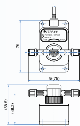
●センサー部取付状態
