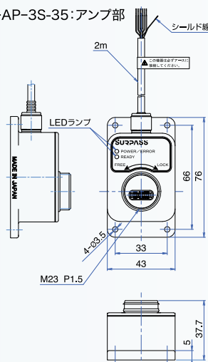
●DTFZ-AP-3S-35:アンプ部
