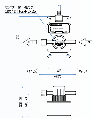
●センサー部取付状態
