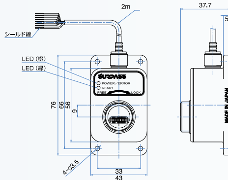
●DTFZ-AP-25: アンプ部
