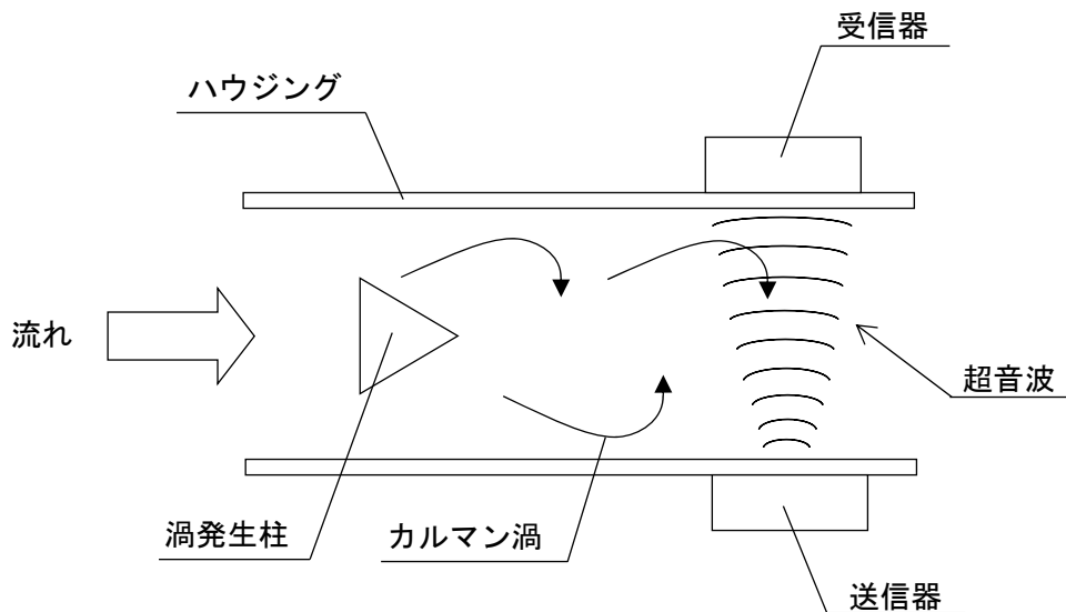
測定原理図
