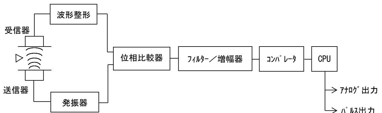
回路構成図
