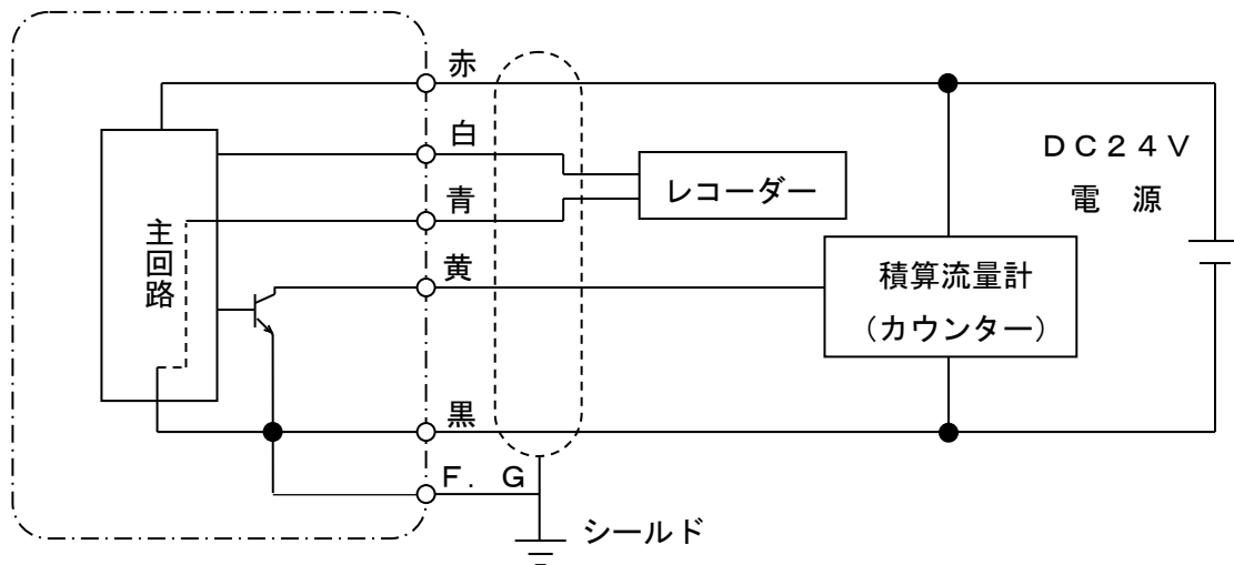
配線図
